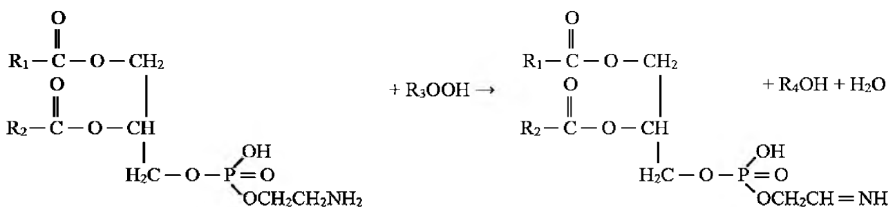
Рисунок 1. Скелет иминовых связей
